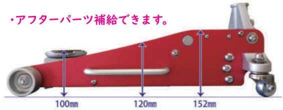
ダブルピストンで上昇時間短縮
